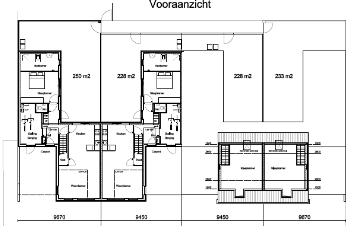
Begane Grond
