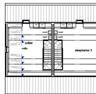
2e Verdieping
