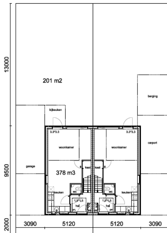
Begane Grond
