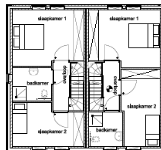
2e Verdieping
