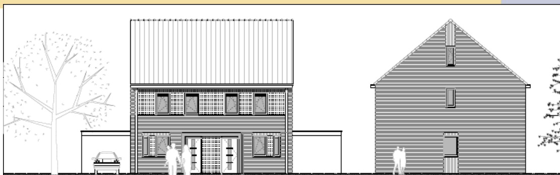
Voorgevel
